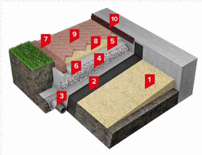
Рис. 3. Пример конструкции мягкой неутепленной отмостки, связанной с системой поверхностного водоотвода.
