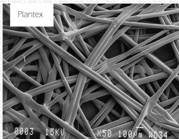
Фото 5. Микроструктура пор геотекстиля Turar SF27, применяемого на мембране PLANTER Geo.
